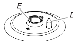
A. Chapeau de brûleur B. Ouverture du tube d'arrivée de gaz C. Base du brûleur D. Électrode d'allumage E. Porte-gicleur
